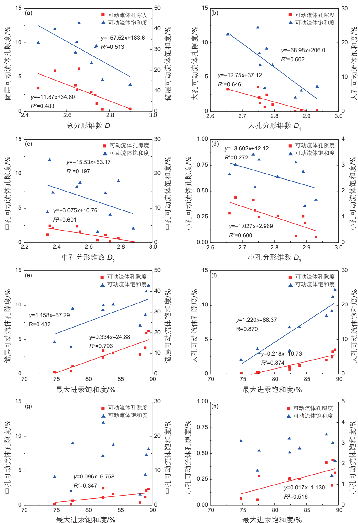
图 10 不同尺寸孔喉内部可动流体孔隙度及饱和度与分形维数和最大进汞饱和度的关系
