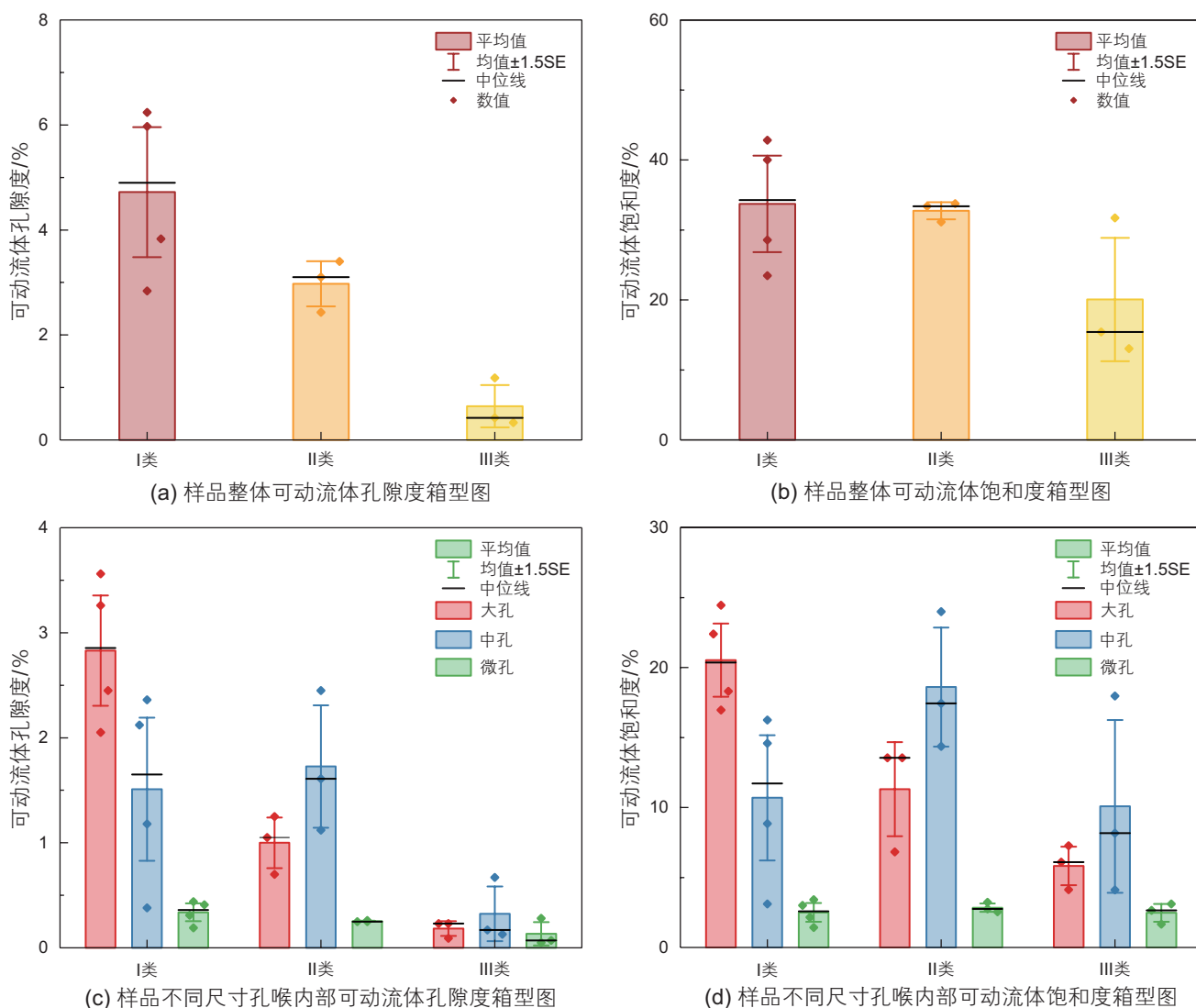
图 11 不同孔喉类型及孔喉尺寸内部可动流体参数分布箱型图
